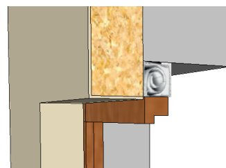
Coffre de volet intégré à la fenêtre
