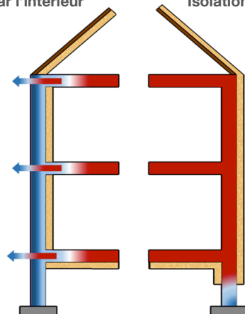
Traitement des ponts thermiques
