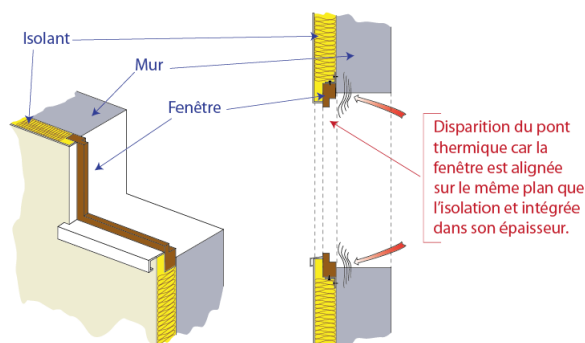
Pose en applique extérieure
