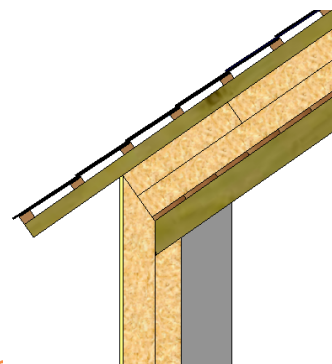
Jonction mur-toiture en isolation par l'extérieur
