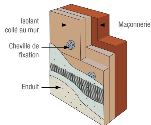
Isolant collé-chevillé et enduit
