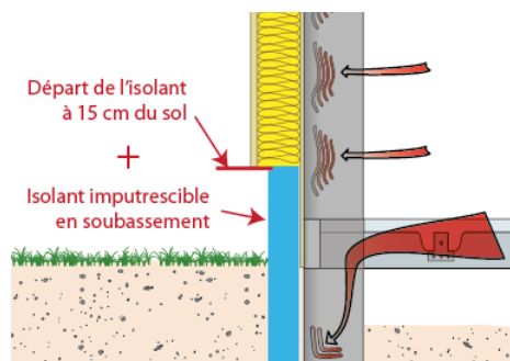
Isolation du soubassement (enterrée)
