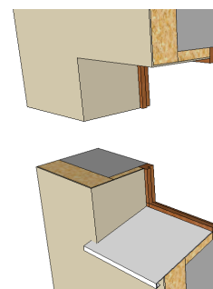
Retour d'isolant sur fenêtre
