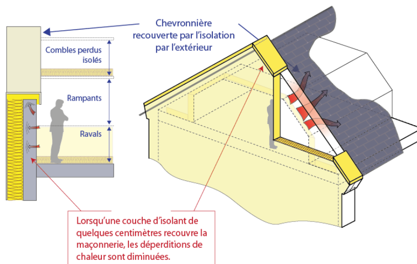
Isolation des chevronnières
