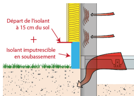
Isolation du soubassement
