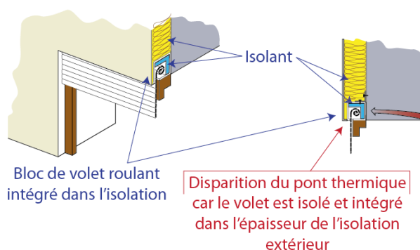
Coffre de volet dans l'épaisseur de l'isolant
