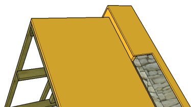
Isolation des chevrons
