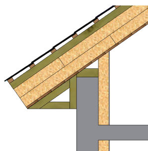
Jonction mur-toiture en cas d'isolation des murs par l'intérieur
