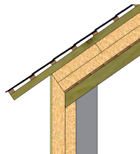
Jonction mur-toiture en cas d'isolation des murs par l'extérieur
