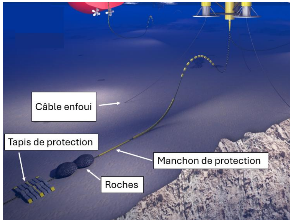
Figure 1-8- Formes de protection d'un câble sous-marin [adapté de Tekmar, 2024]
