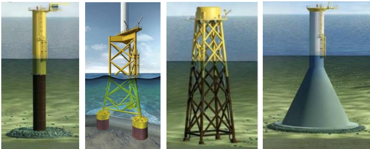
Figure 1-9: Types de fondations éoliennes en mer posées sur le fond marin (de gauche à droite : monopieu, jacket avec ancrage à succion, jacket à pieux, fondations gravitaires) [Dührkop et al., 2016 ; Sparrevik, 2019]
