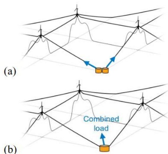
Figure 4-2 : (a) ancrées individuelles et (b) remplacement des paires d'ancres par des ancres partagées [Hall et al., 2022]
