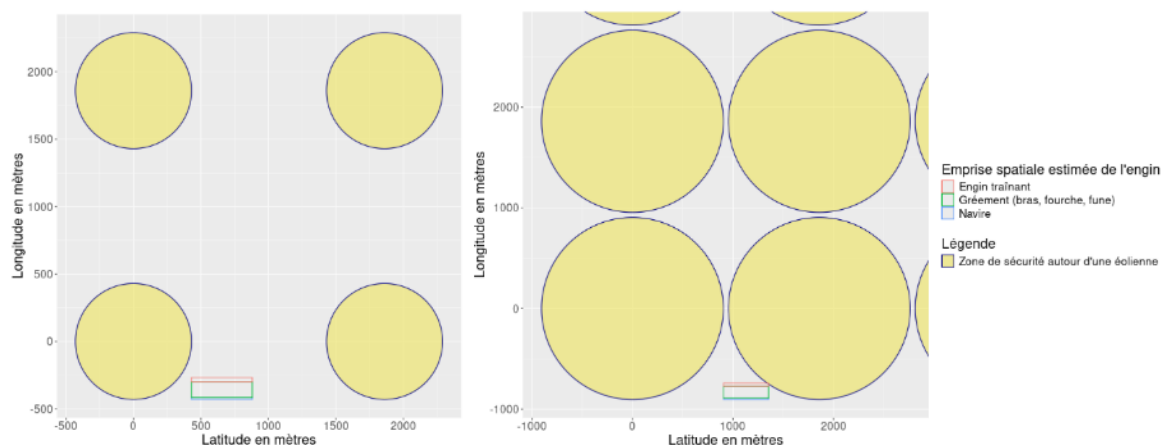
Figure 3-2- Représentation graphique d'une course de 450 mètres d'un chalutier de fond, éolien flottant 25MW – profondeur 95 m – ancrage semi-tendu à gauche / gravitaire à droite.
