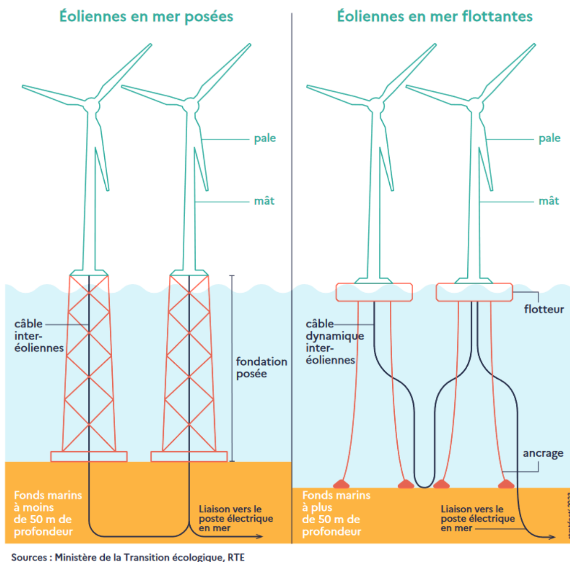
Figure 1-1 : Composants principaux d'une éolienne en mer posée (gauche) et flottante (droite) [Eoliennes en mer en France, 2024]
