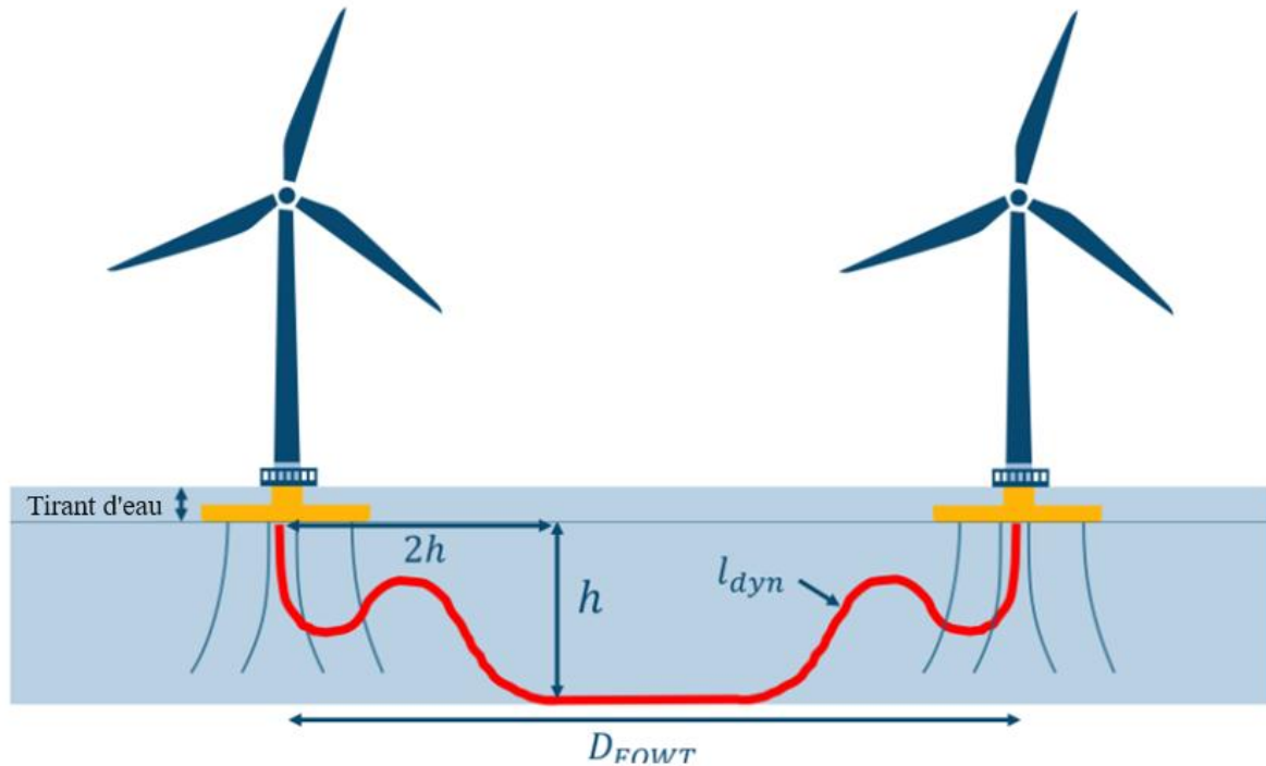
Figure 1-22 : Câble inter-réseaux reliant deux éoliennes flottantes
