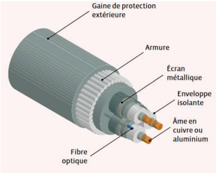
Figure 1-3 : Section transversale d'un câble d'exportation [RTE, 2023]
