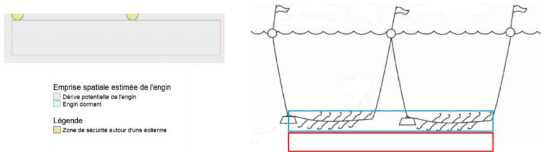
Figure 2-6 - Représentation de l'emprise spatiale de l'engin pour la palangre. Adapté de [https://www.researchgate.net/figure/The-Gulf-of-Gab-s-location-of-bottom-longline-sets-Stars-sets-of-class-I-w_fig1_257614775]
