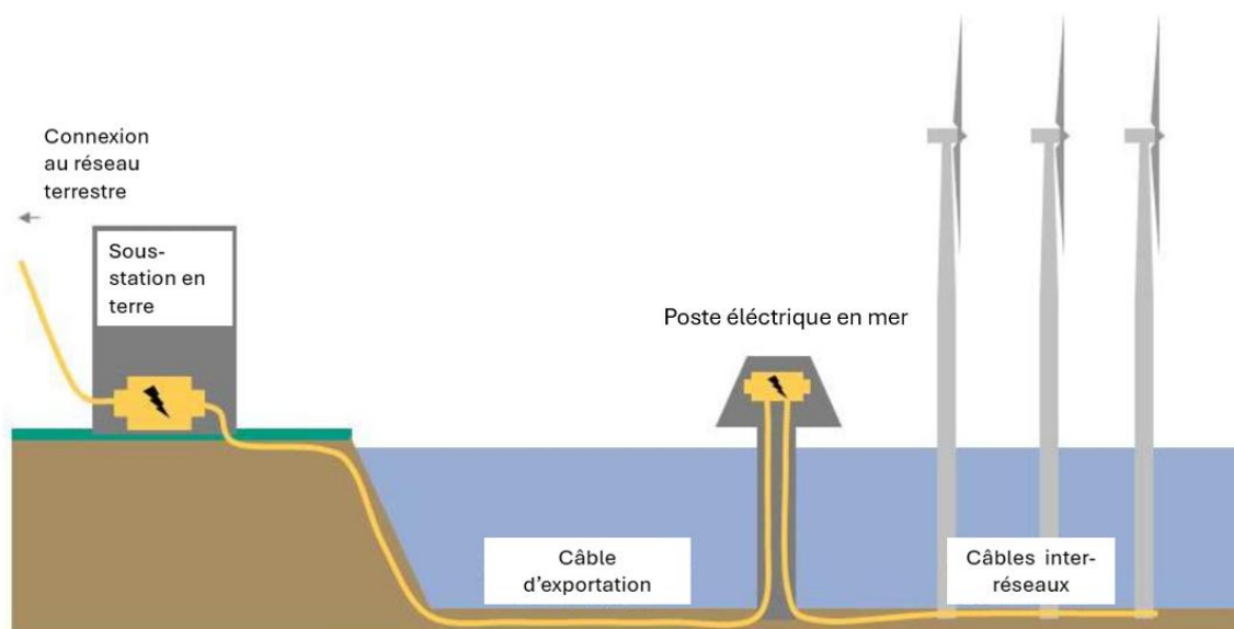
Figure 1-1 : Composants de transmission d'un parc éolien en mer typique [adapté de Catapult, 2015]
