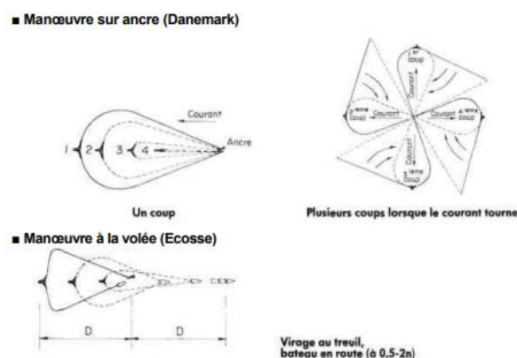
Figure 2-7 - Différentes manœuvres de sennes de fond [FAO, 1988]
