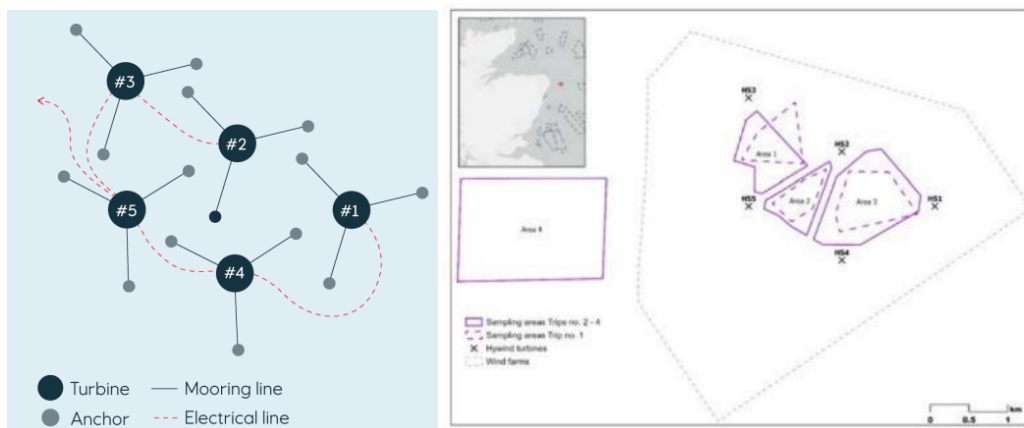
Figure 3-6 : Configuration du parc de Hywind [Equinor] et localisation des zones d'essai [Wright et al., 2023]
