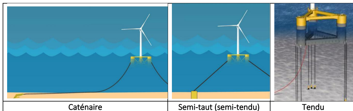
Figure 1-18 : Systèmes d'ancrage de l'éolien flottant [BVG Associates, 2023 ; Renewables, 2022]
