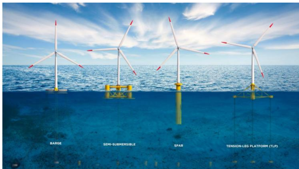
Figure 1-15: Types de flotteurs d'éoliennes flottantes [Green Giraffe, 2017]
