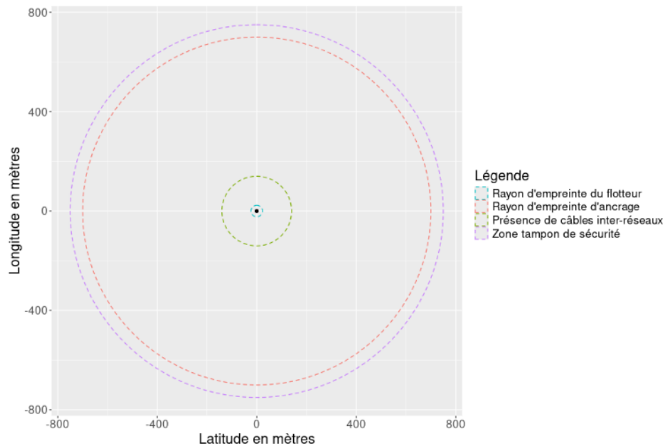
Figure 2-1 – Schéma d’une zone d’exclusion recommandée en matière de sécurité maritime autour d’une éolienne dans l’outil COPEOLE
