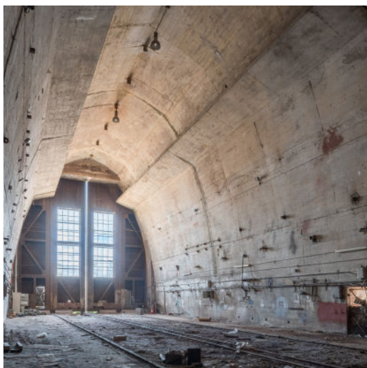
Dom-bunker ouest dit «T6».
